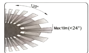
Distância de detecção: Max.10Mt
